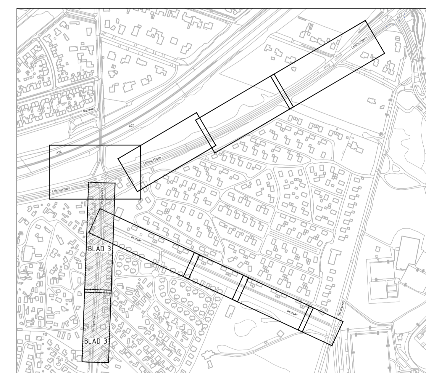
OVERZICHTSTEKENING
